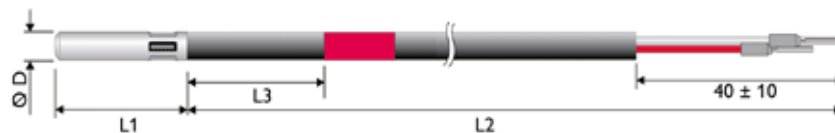
Cuadro sinóptico Pt1000 - FKP5,5 / FRP5,5
